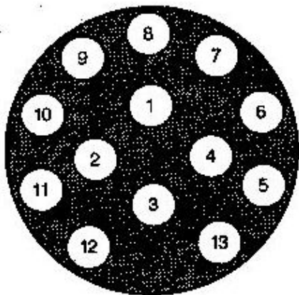
Kontaktbelegung des Steckers
